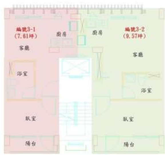
3樓平面配置圖
